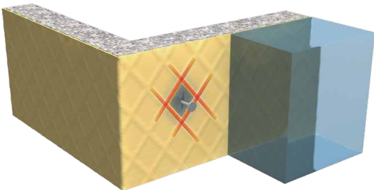
Detalle de penetración de tuberías con SikaProof® Tape-150
